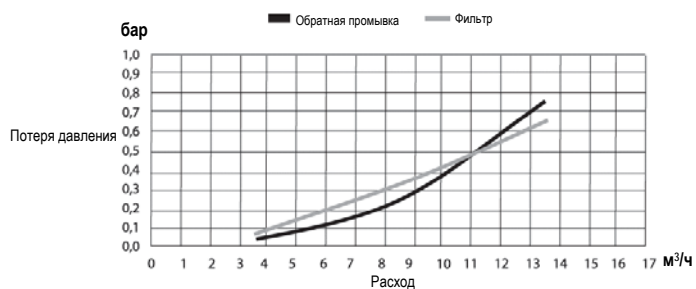
Клапан 1 1/2"
