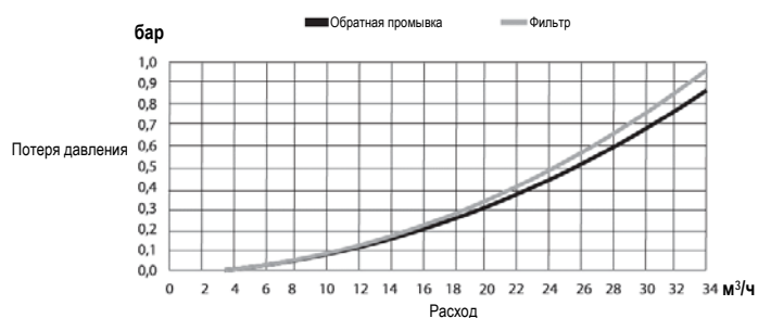
Клапан 2"
